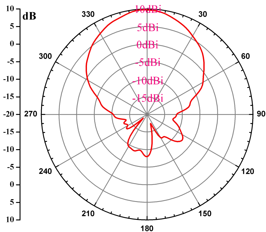
图 5 E 面二维方向图
